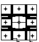
جزئیات نبش اتصال ستون به صفحه
