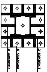
جزئیات نبش اتصال ستون به صفحه
